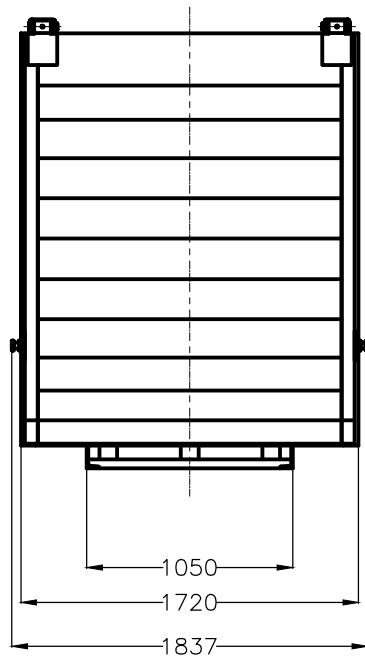
Vista trasera
