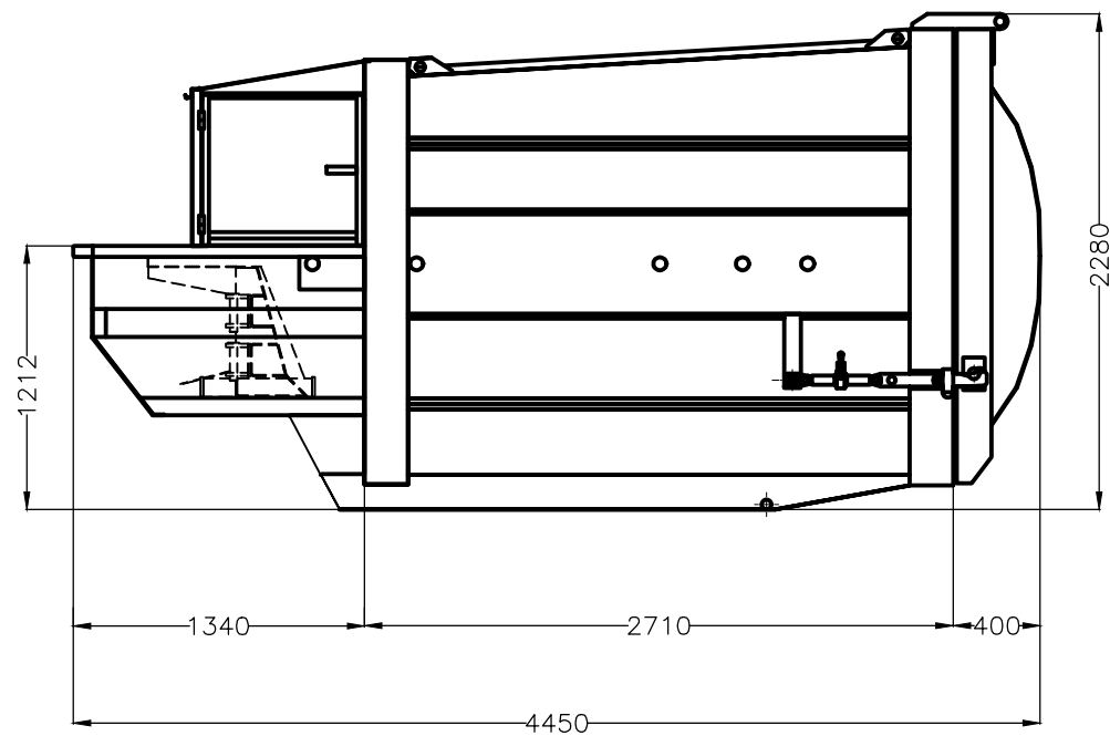
Vista lateral
