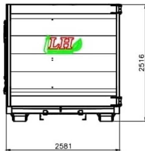
VISTA TRASERA
