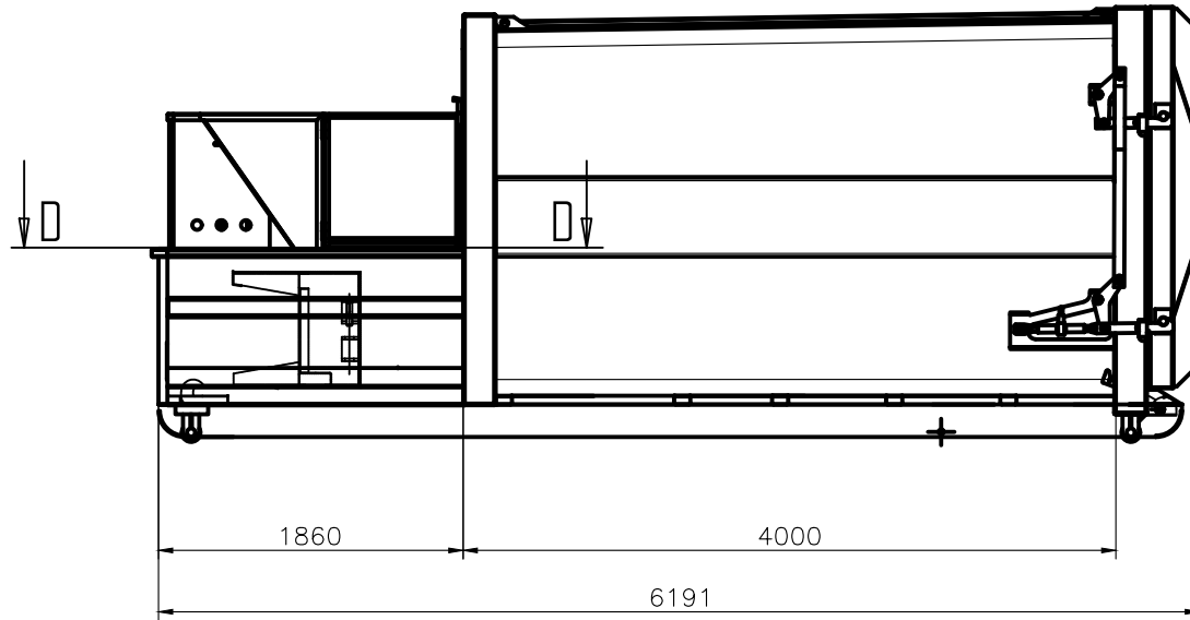
VISTA LATERAL
