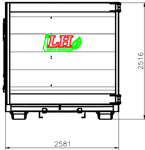
VISTA TRASERA
