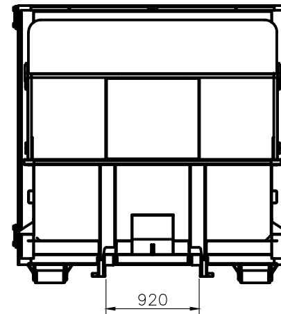
VISTA DELANTERA
