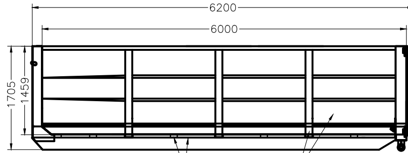
Travesaños de piso 1/8" Piso en chapa espesor 3/16"
