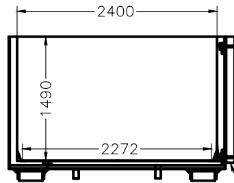
Puerta en chapa 2.5mm Marco inferior 100x100 espesor 3.2mm
